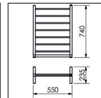
19.TQ13.IP PISO
