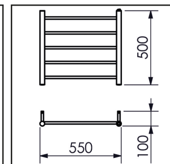
19.TY01.IP PEQUENO FIO APARENTE
