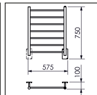
19.TY04.IP GRANDE FIO OCULTO
