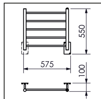
19.TY02.IP PEQUENO FIO OCULTO
