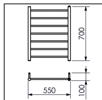
19.TY03.IP GRANDE FIO APARENTE
