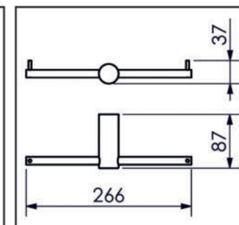
03.SG00.CR PAPELEIRA DUPLA
