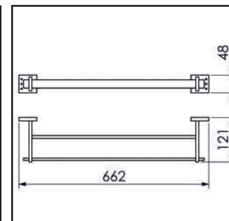
60CM 09.TB02.CR TOALHEIRO DUPLO
