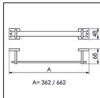
30CM 07.TB02.CR 60CM 07.TB04.CR TOALHEIRO
